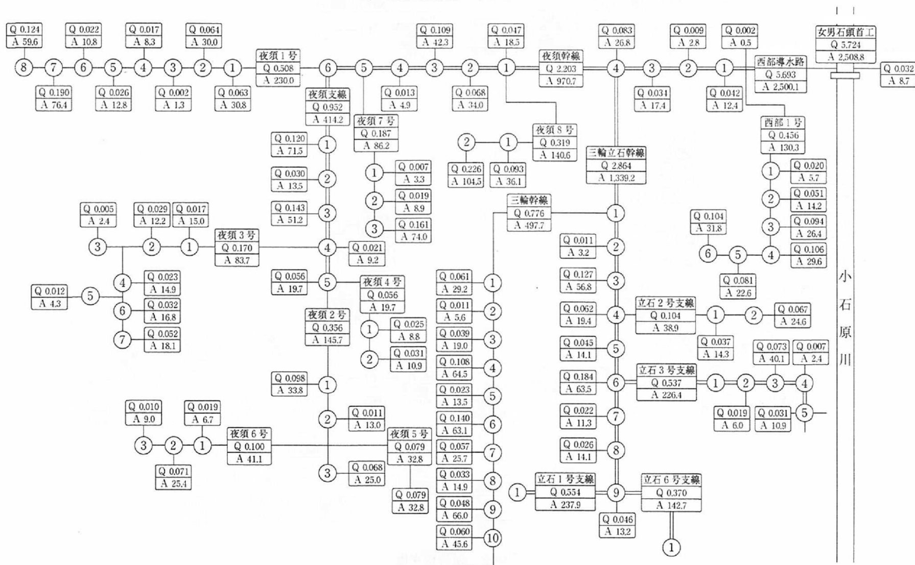
用水系統図 その3
