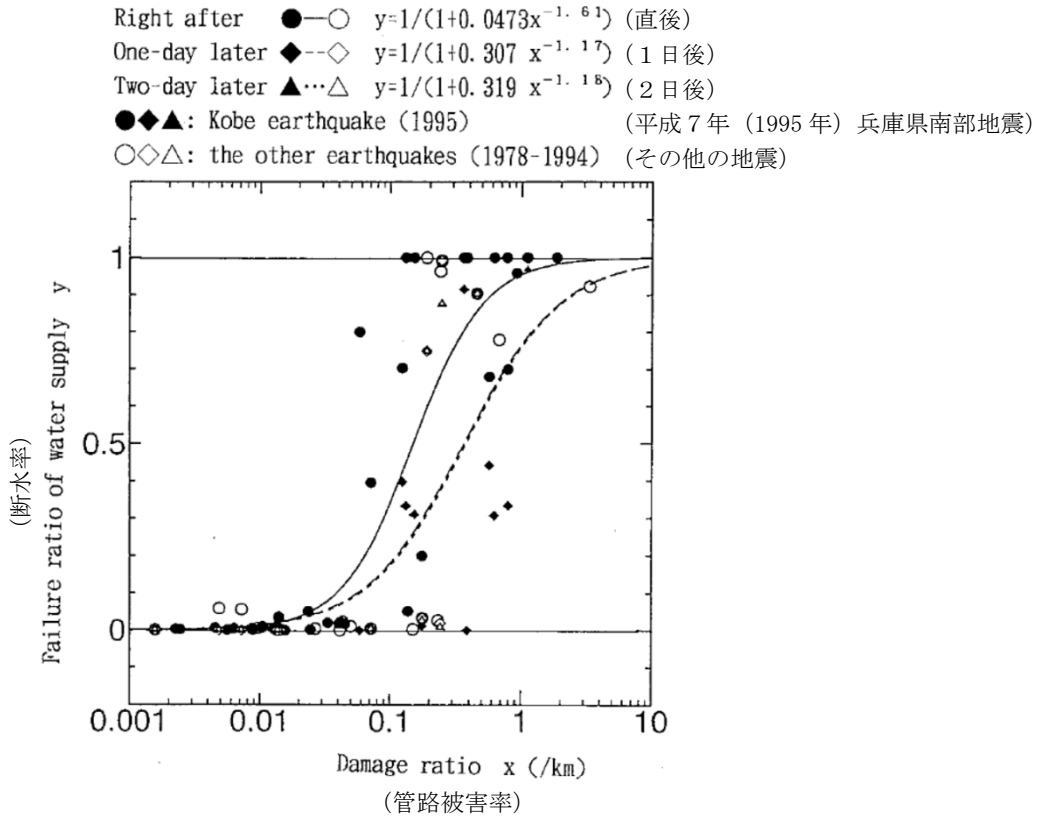
図Ⅲ.3-4 川上式による管路被害率と断水率の関係 (川上(1996))
