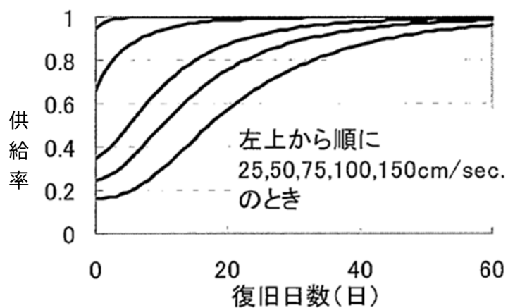
図Ⅲ.3-8 下水道の供給率曲線
