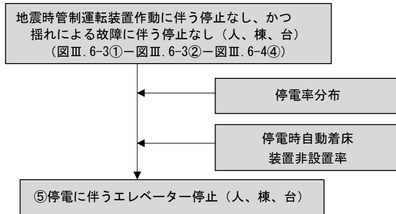
図Ⅲ.6-5 地域の停電に伴うエレベーター停止想定フロー (内閣府 (2025) )
