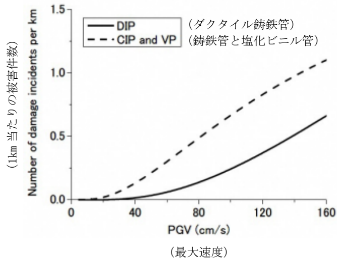
図Ⅲ. 3-5 送水管・配水管の被害率関数 (丸山ら(2010))
