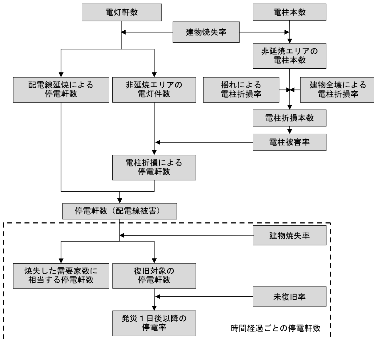
図Ⅲ. 3-1 電力被害想定フロー（内閣府（2025）を基に作成）
