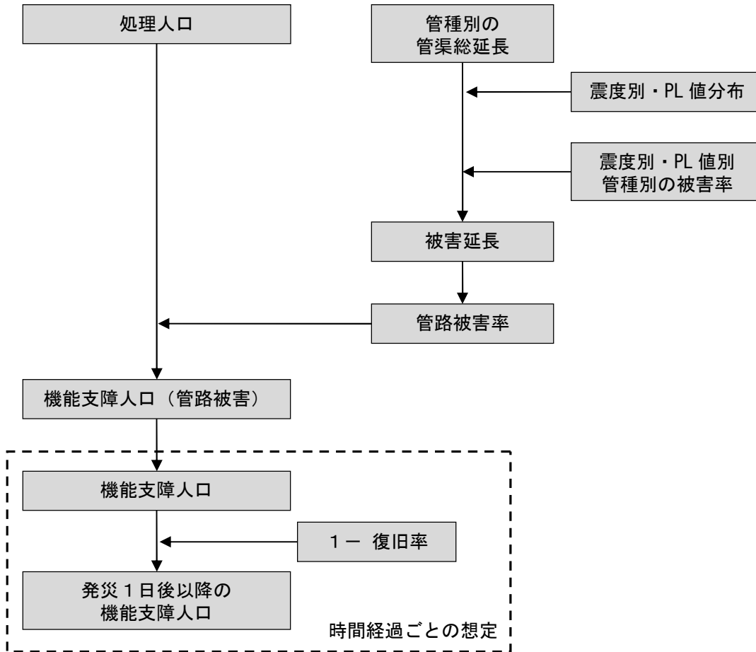
図Ⅲ.3-7 下水道被害想定フロー(内閣府(2025)を基に作成)
