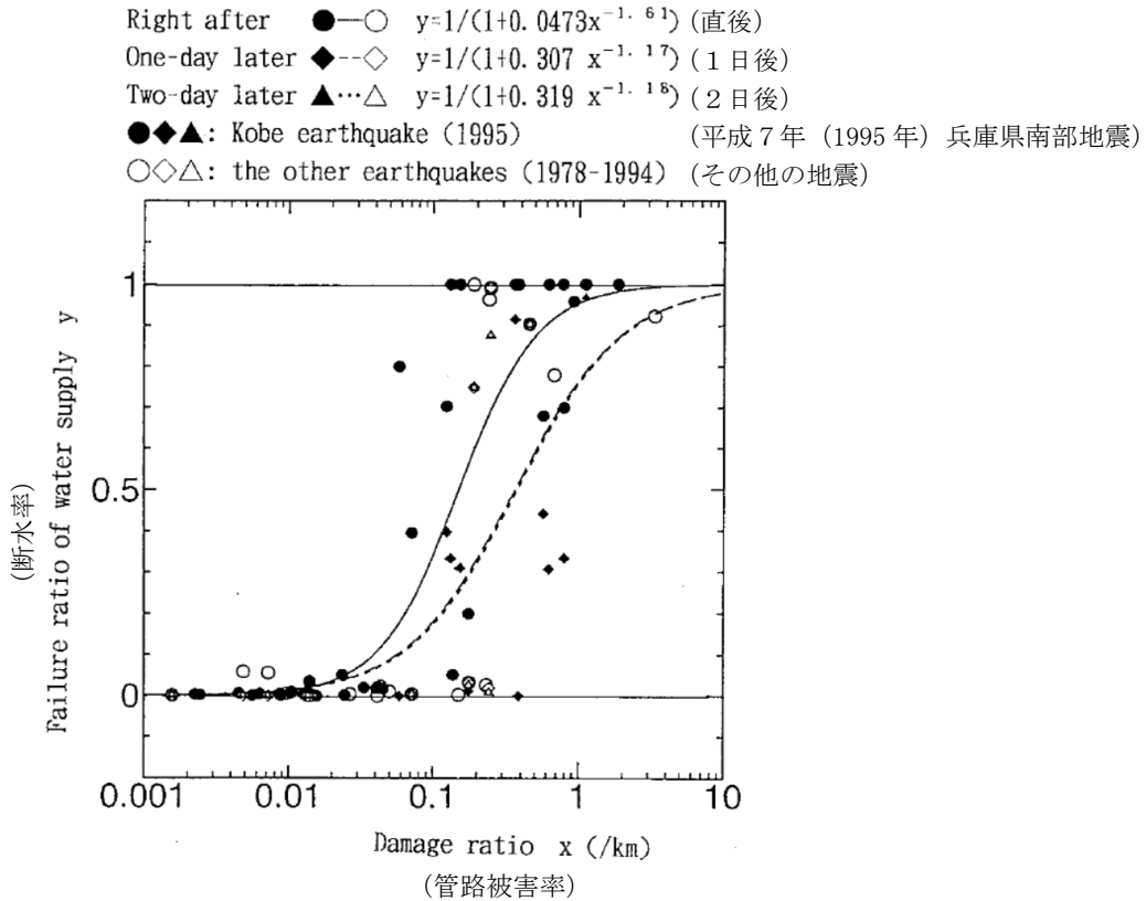
図 3-4 川上式による管路被害率と断水率の関係 (川上 (1996) )
