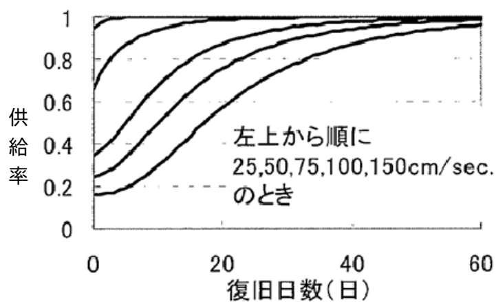
図Ⅲ.3-8 下水道の供給率曲線
