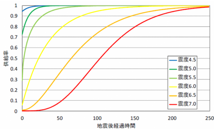
図Ⅲ.3-2 計測震度に対する供給率曲線(電力供給率曲線)
