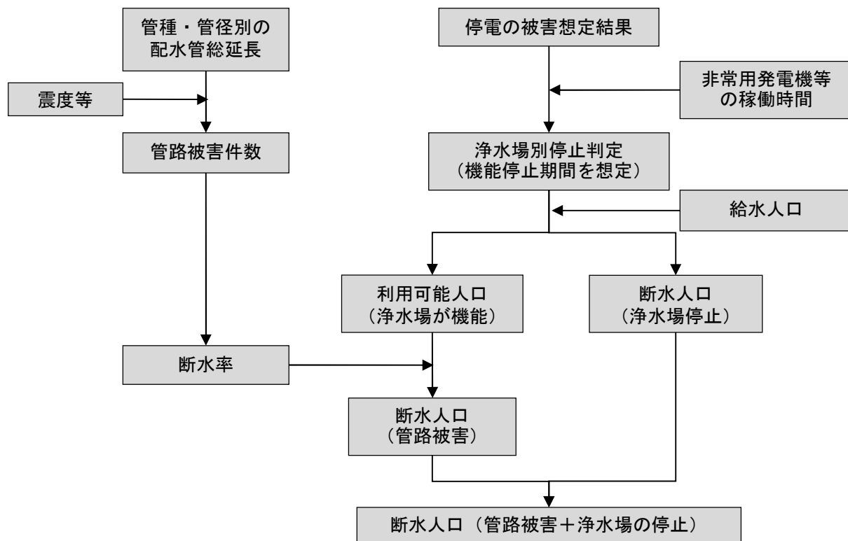
図Ⅲ.3-3 上水道被害想定フロー (内閣府(2025)を基に作成)
