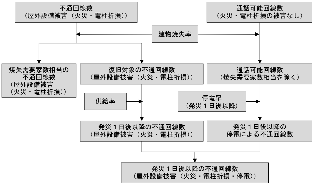
図Ⅲ. 3-10 固定電話通信被害復旧想定フロー (内閣府 (2025) を基に作成)
