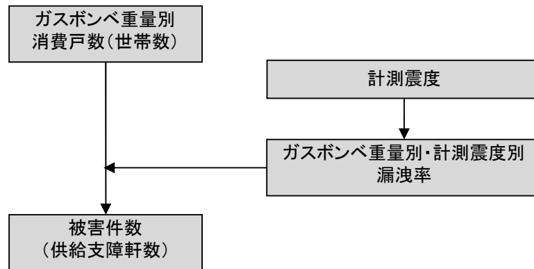
図Ⅲ.3-15 LP ガスの被害想定フロー (関沢ら (2003) を基に作成)
