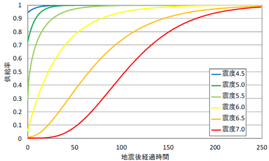
図Ⅲ.3-12 計測震度に対する供給率曲線(電力) (再掲)
