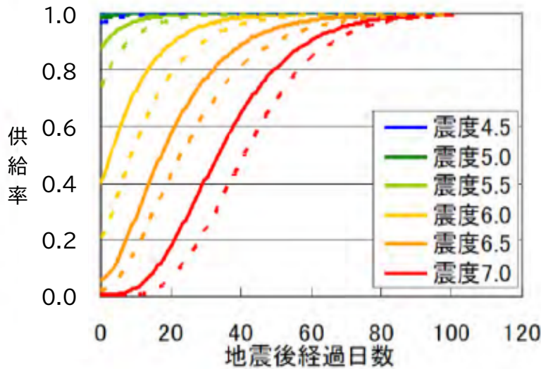
図Ⅲ.3-6 上水道の供給率曲線(破線:オリジナル、実線:改良モデル)
