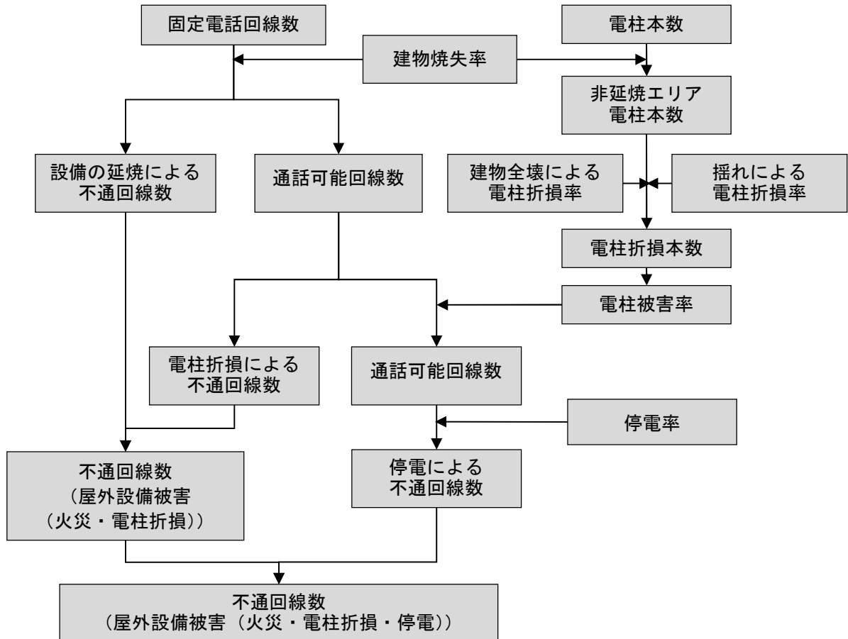
図Ⅲ.3-9 固定電話通信被害想定フロー（内閣府（2025）を基に作成）
