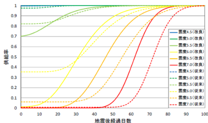
図Ⅲ.3-14 都市ガスの計測震度に対する供給率曲線
