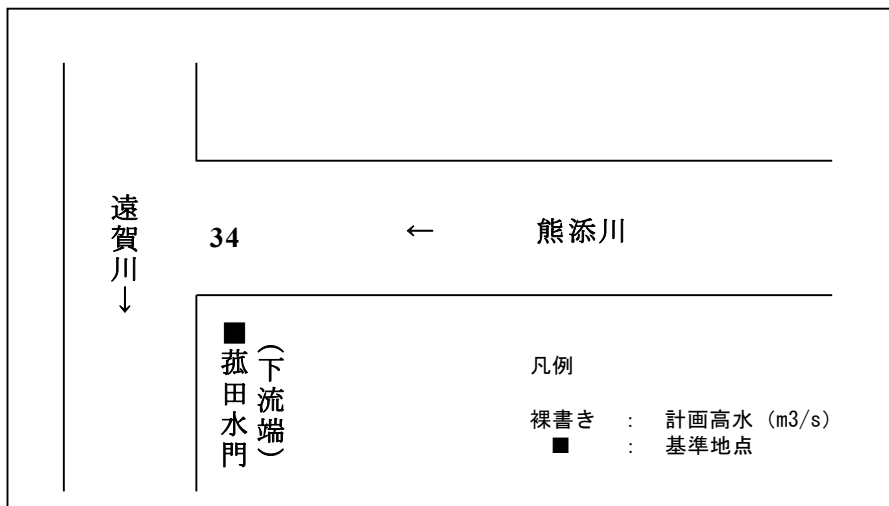
図 3-1(1) 熊添川計画流量配分図
