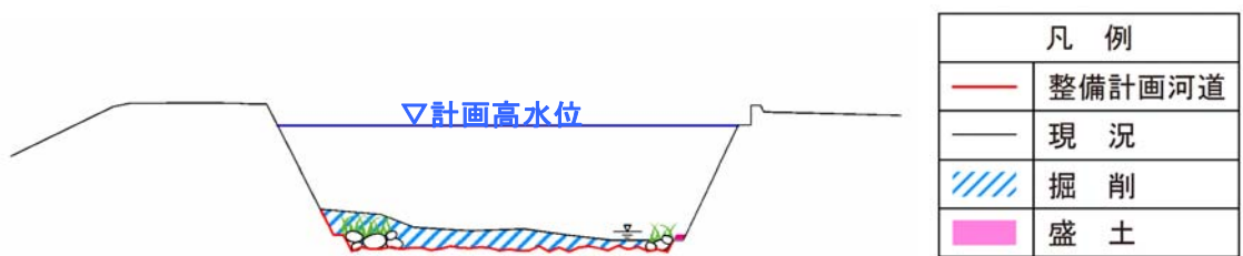
図 4-5(2) 建花寺川河川整備計画代表横断面図(日新橋付近)
