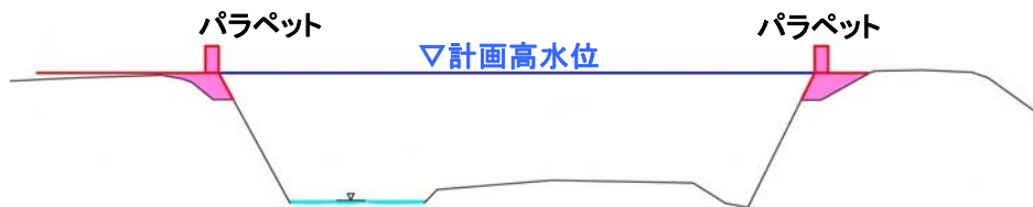
図 4-5(1) 建花寺川河川整備計画代表横断面図(ツゲノ木井堰下流区間)
