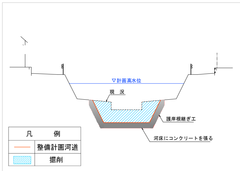
図 4-3 熊添川河川整備計画代表横断図
