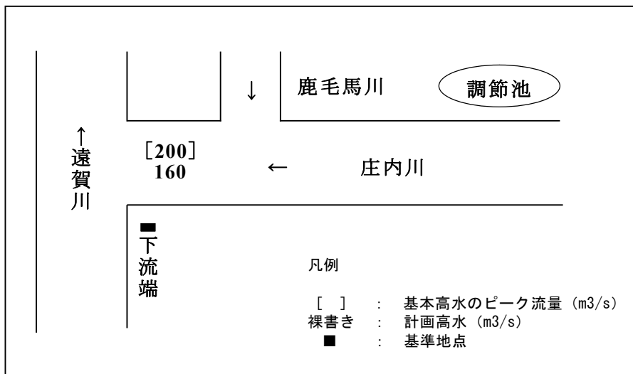
図 3-1(4) 庄内川計画流量配分図
