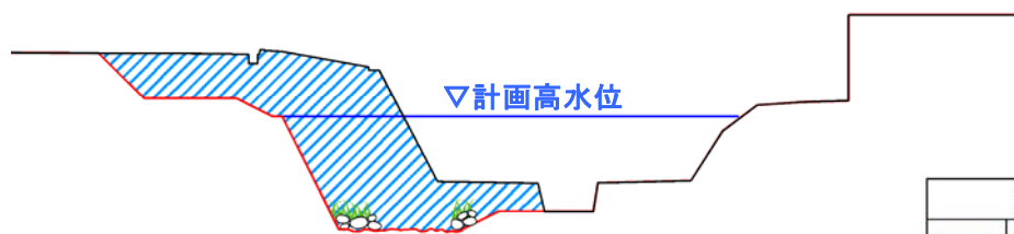
図 4-7(1) 庄司川河川整備計画代表横断図(下流区間)
