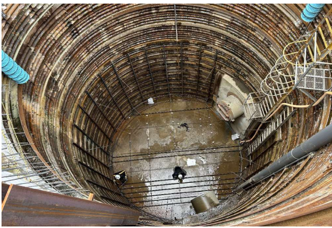
施工状況（分土工3工区）
