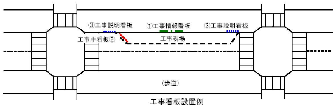
標示板の設置場所
