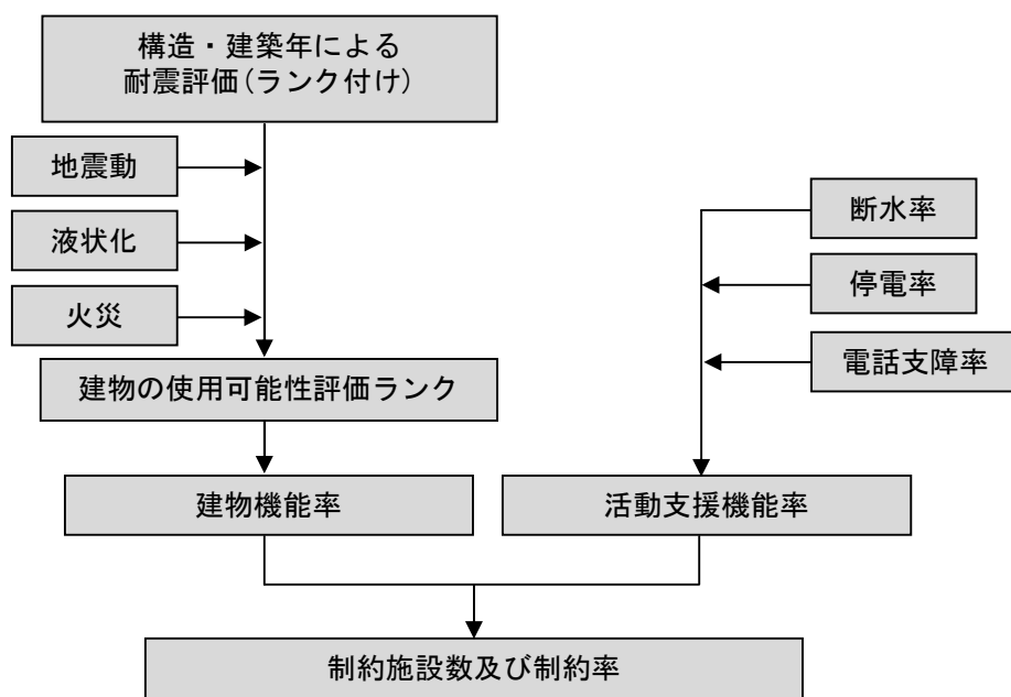
図Ⅲ. 5-1 重要施設被害想定フロー
