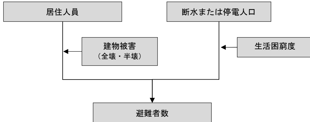
図Ⅲ.2-14 避難者数（発災直後）算出フロー（内閣府（2025）を基に作成）
