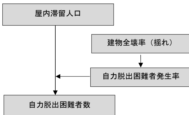
図Ⅲ. 2-13 揺れによる建物被害に伴う要救助者の想定の流れ（内閣府（2025）を基に作成）
