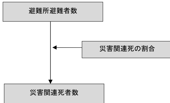
図Ⅲ.2-15 災害関連死者数の想定の流れ（内閣府（2025）を基に作成）
