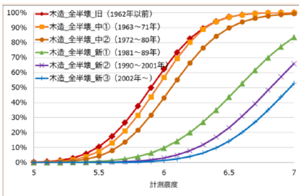
木造建物の全半壊率曲線
