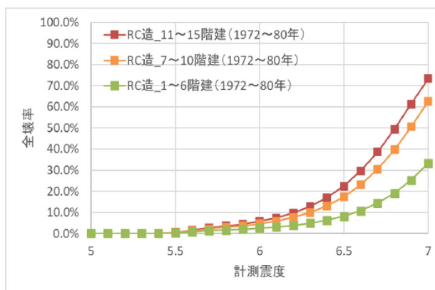
RC・SRC造（1972～80年以前）の全壊率曲線
