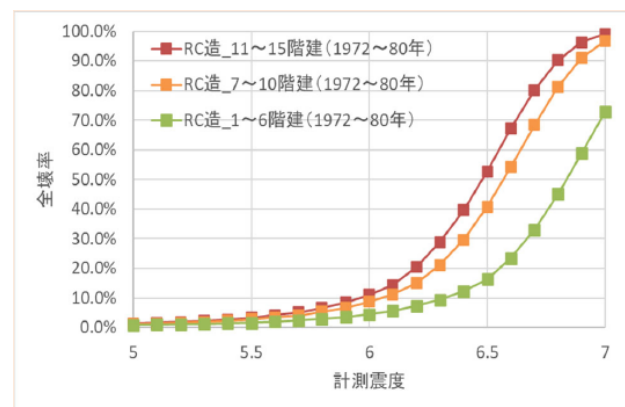
RC・SRC造（1972～80年以前）の全半壊率曲線
