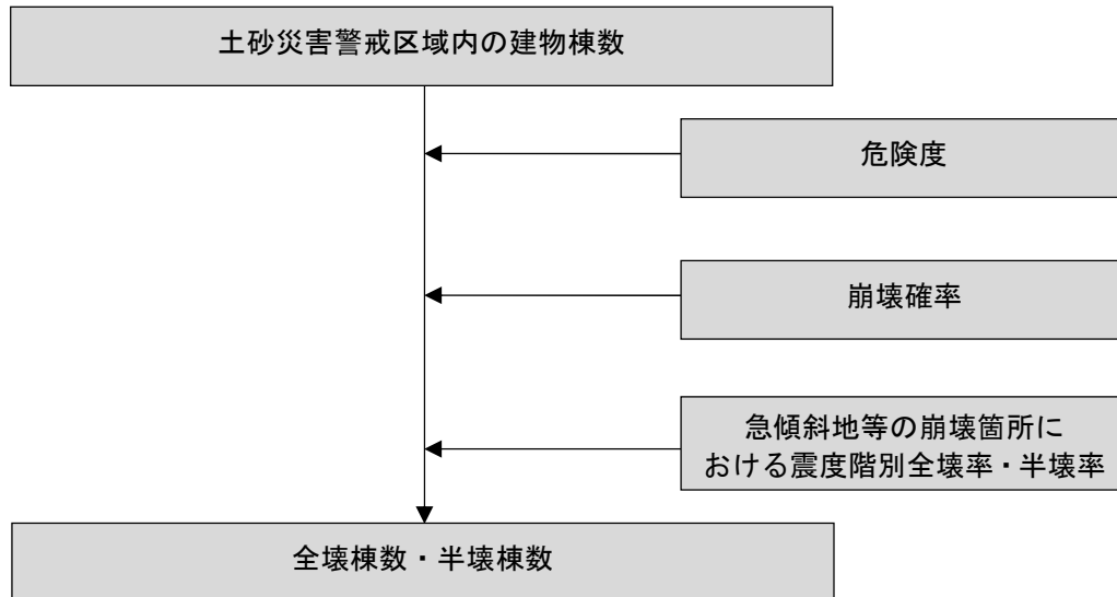
図Ⅲ. 1-11 急傾斜地崩壊による建物被害算定フロー（内閣府（2025）を基に作成）
