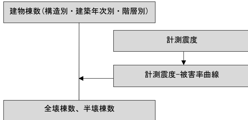
図Ⅲ.1-8 揺れによる建物被害算定フロー（内閣府（2025）を基に作成）
