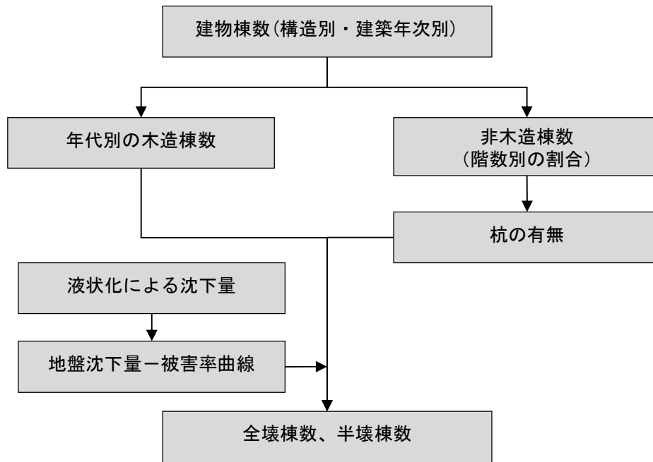
図Ⅲ.1-6 液状化による建物被害想定フロー（内閣府（2025）を基に作成）
