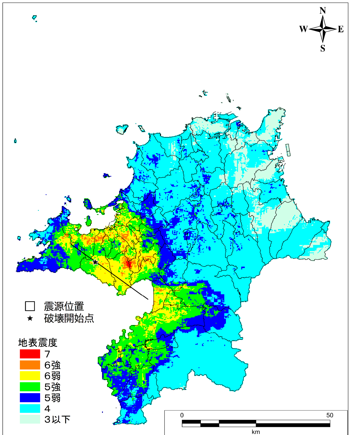
図Ⅱ.2-70 地表震度分布図 【日向峠-小笠木峠断層帯 (破壊開始点：中央)】
