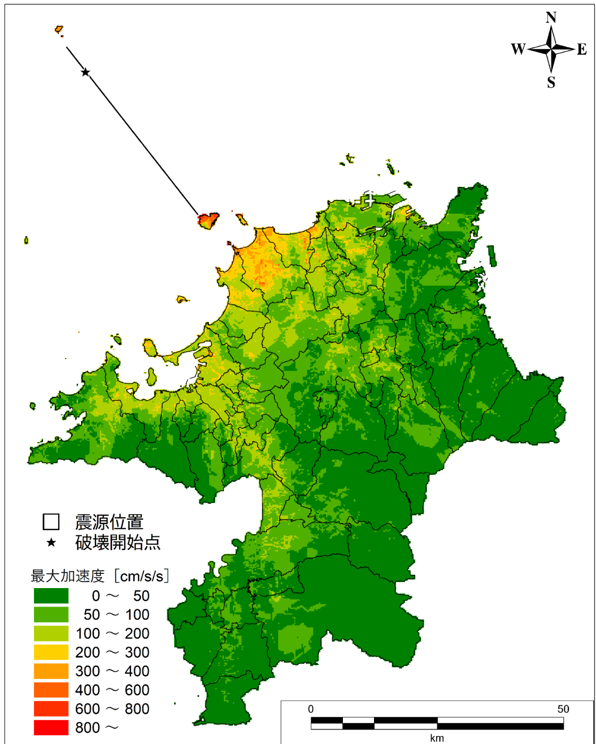
図Ⅱ.2-18 地表加速度分布図 【西山断層帯大島沖区間（破壊開始点：北側）】
