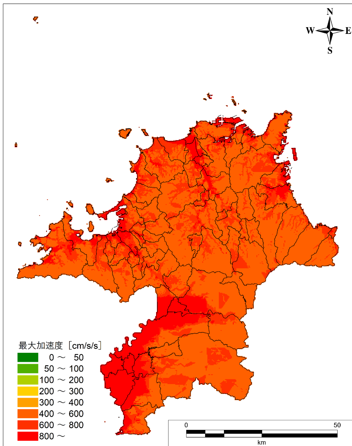
図Ⅱ.2-43 地表加速度分布図
