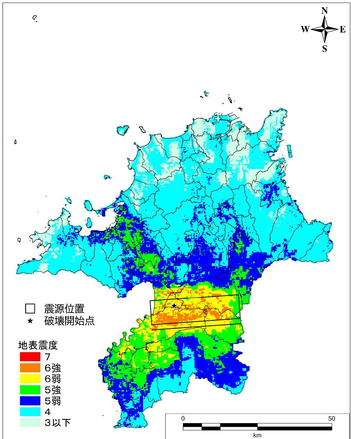
図Ⅱ.2-74 地表震度分布図 【水縄断層帯(破壊開始点：西側)】
