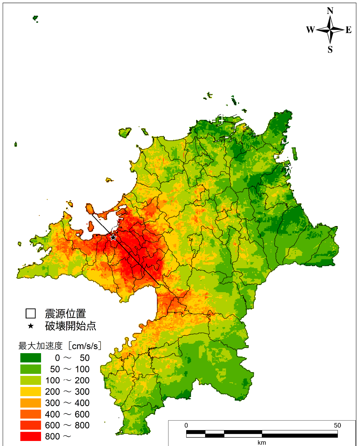
図Ⅱ.2-32 地表加速度分布図 【警固断層帯南東部（破壊開始点：中央）】
