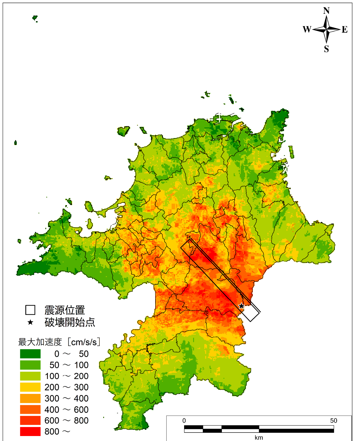
図Ⅱ.2-24 地表加速度分布図 【西山断層帯嘉麻峠区間（破壊開始点：南側）】
