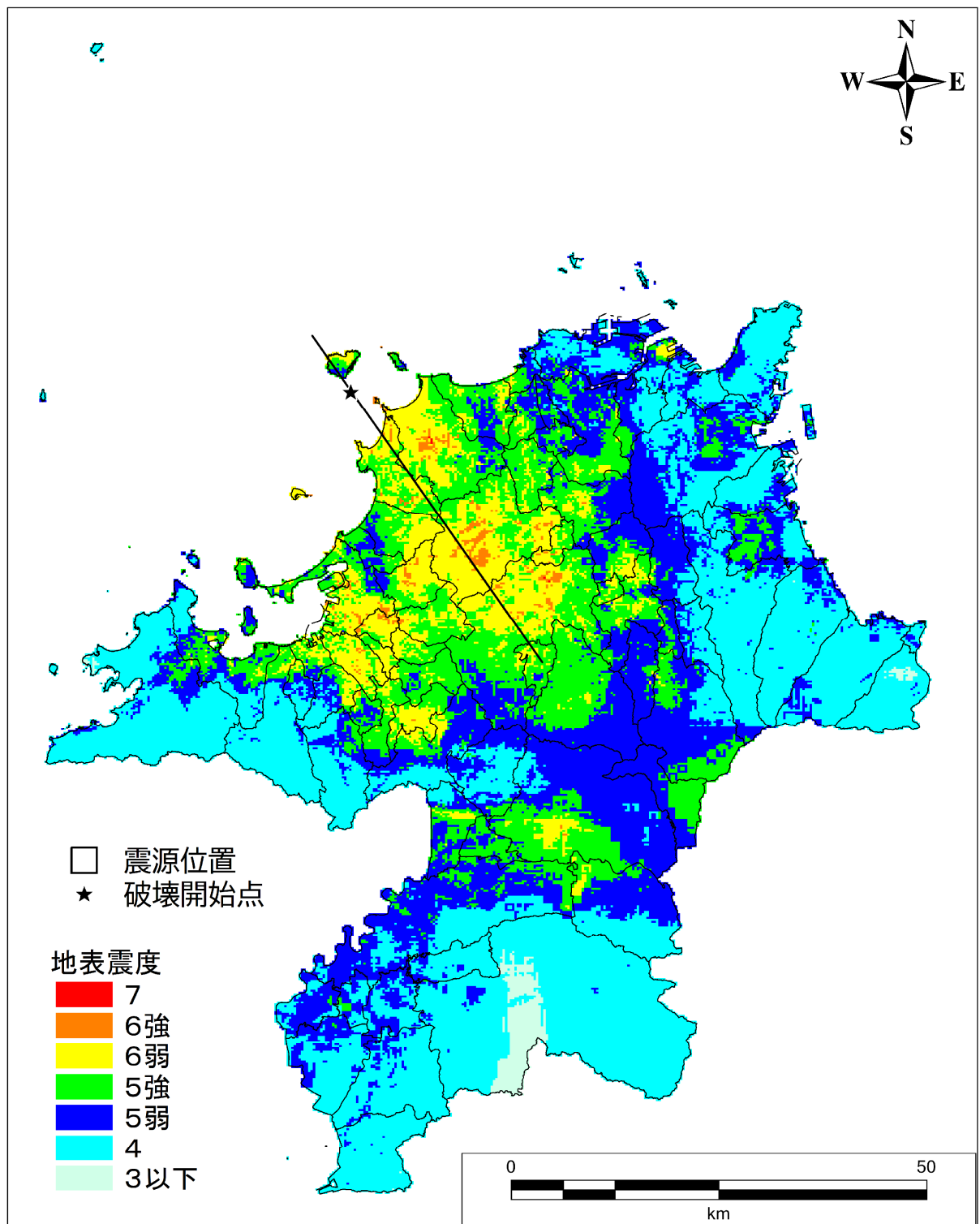
図Ⅱ.2-52 地表震度分布図 【西山断層帯西山区間（破壊開始点：北側）】
