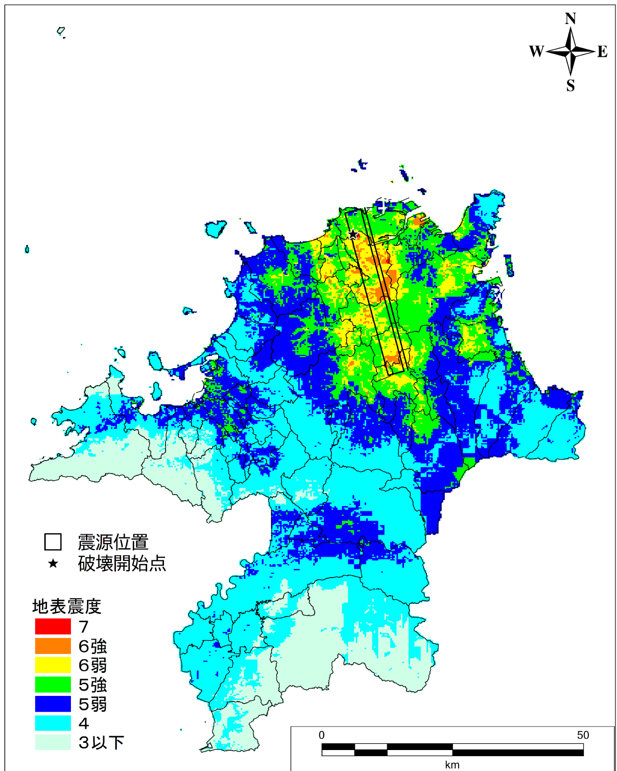
図Ⅱ.2-48 地表震度分布図 【福智山断層帯（破壊開始点：北側）】
