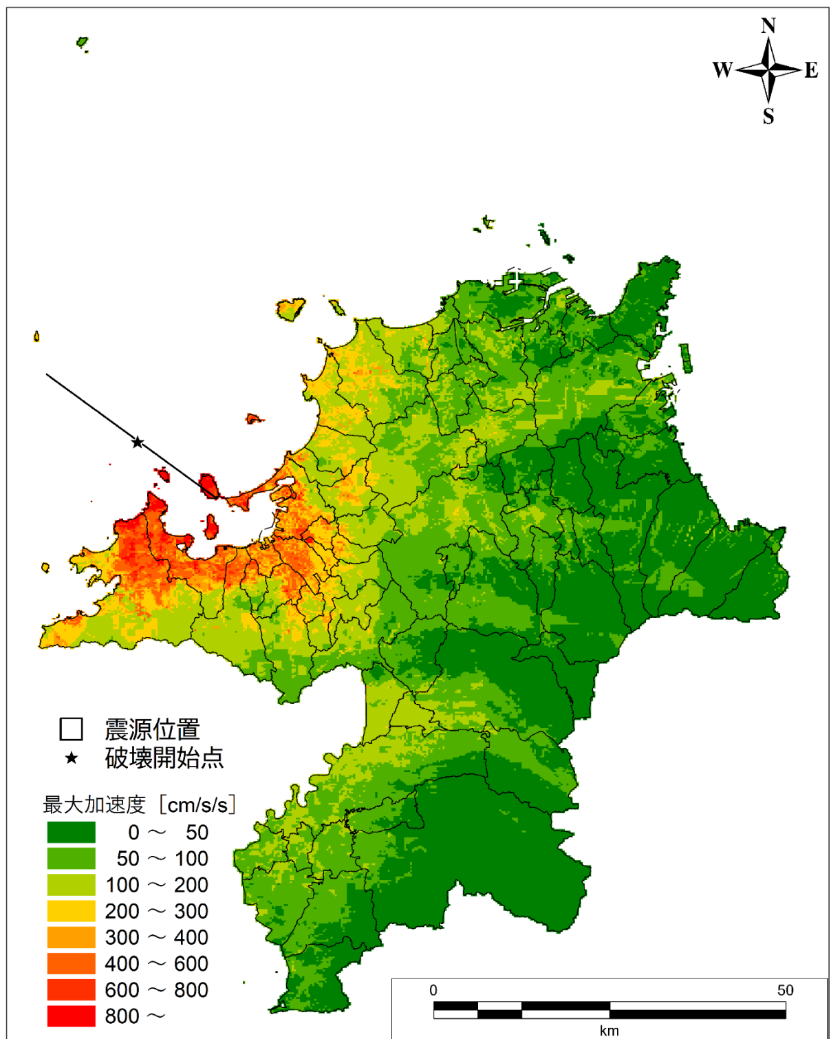
図Ⅱ.2-30 地表加速度分布図 【警固断層帯北西部（破壊開始点：中央）】
