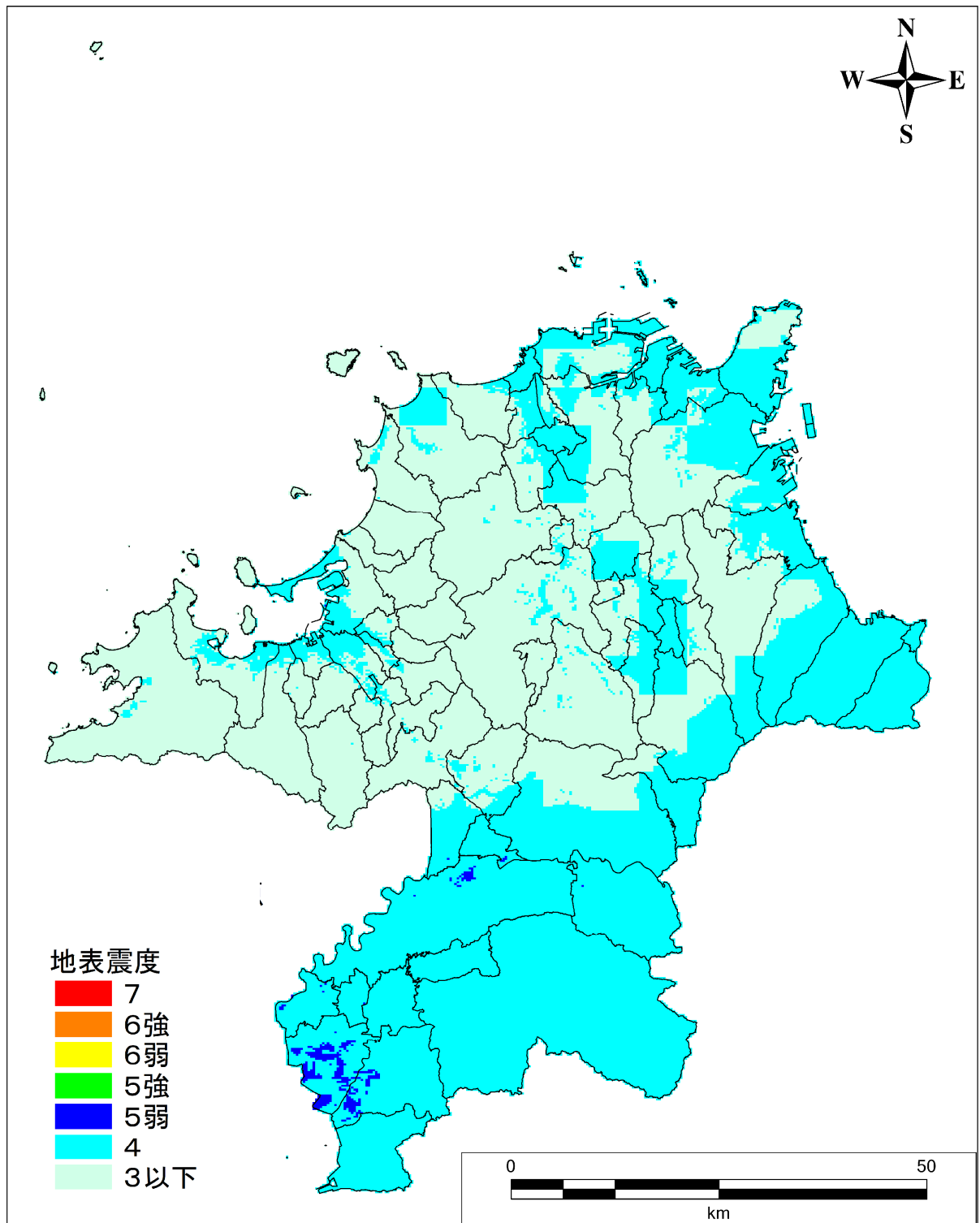
図Ⅱ.2-44 地表震度分布図 【南海トラフ（基本ケース）】
