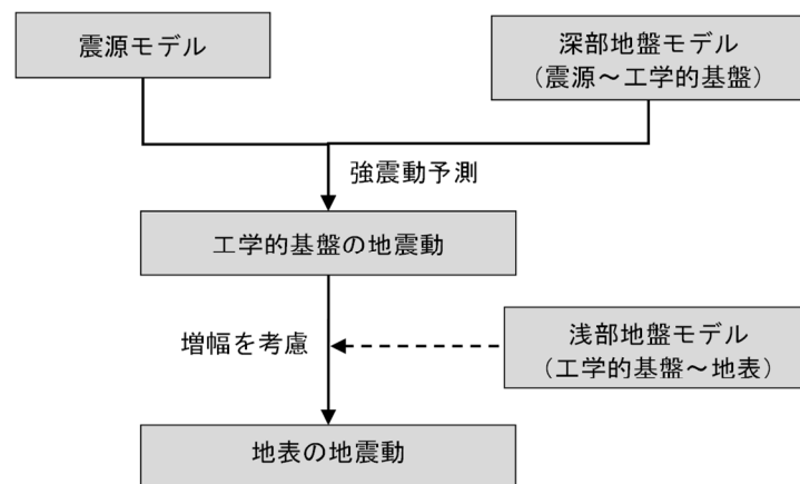
図Ⅱ.2-2 地震動予測の流れ
