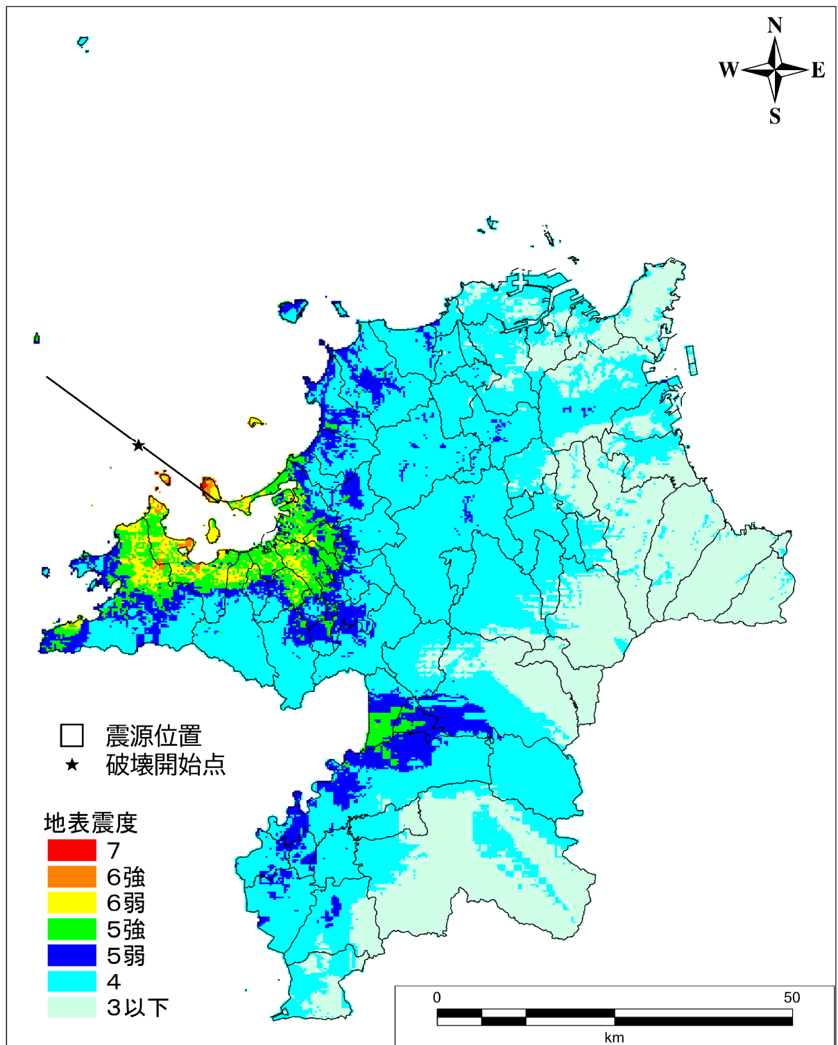
図Ⅱ.2-62 地表震度分布図 【警固断層帯北西部（破壊開始点：中央）】
