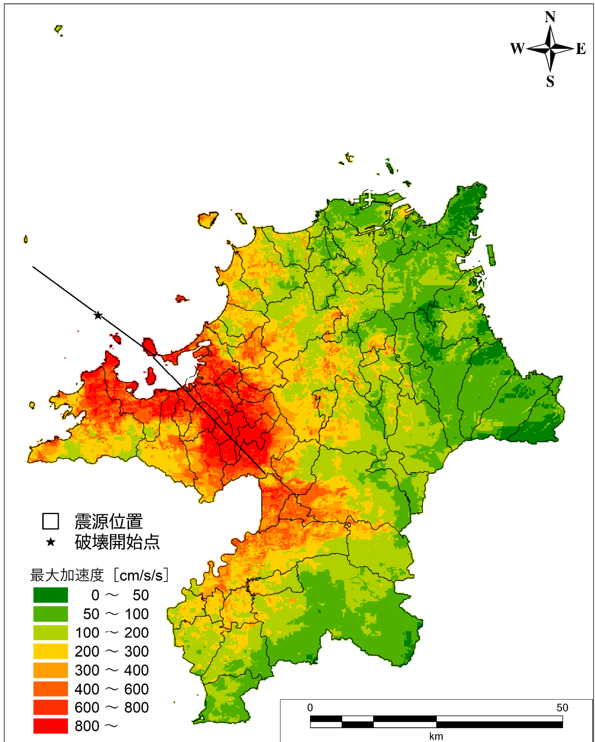
図Ⅱ.2-34 地表加速度分布図 【警固断層帯（北西部+南東部）（破壊開始点：北側）】
