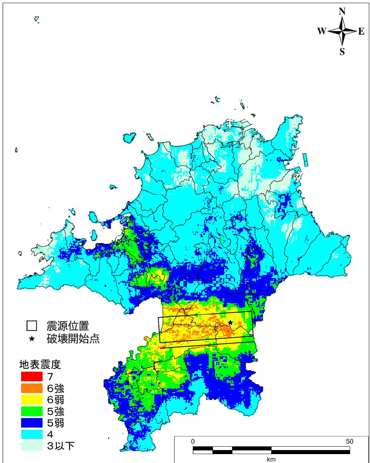
図Ⅱ.2-72 地表震度分布図 【水縄断層帯（破壊開始点：東側）】
