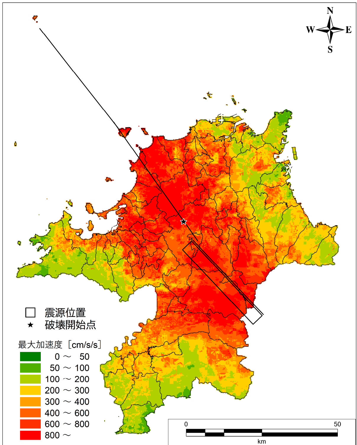
図Ⅱ.2-26 地表加速度分布図 【西山断層帯（大島沖区間＋西山区間＋嘉麻峠区間）（破壊開始点：中央）】
