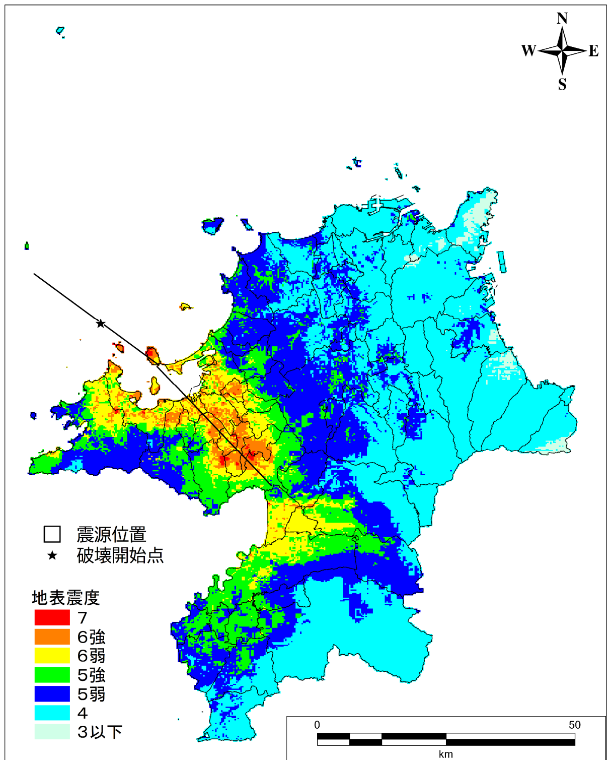
図Ⅱ.2-66 地表震度分布図 【警固断層帯（北西部＋南東部）（破壊開始点：北側）】
