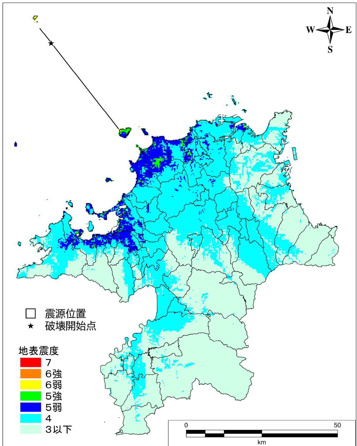
図Ⅱ.2-50 地表震度分布図 【西山断層帯大島沖区間（破壊開始点：北側）】
