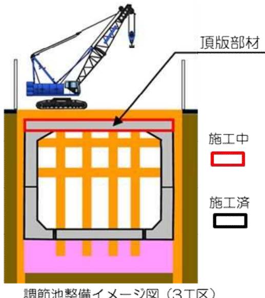
調節池整備イメージ図（3工区）
