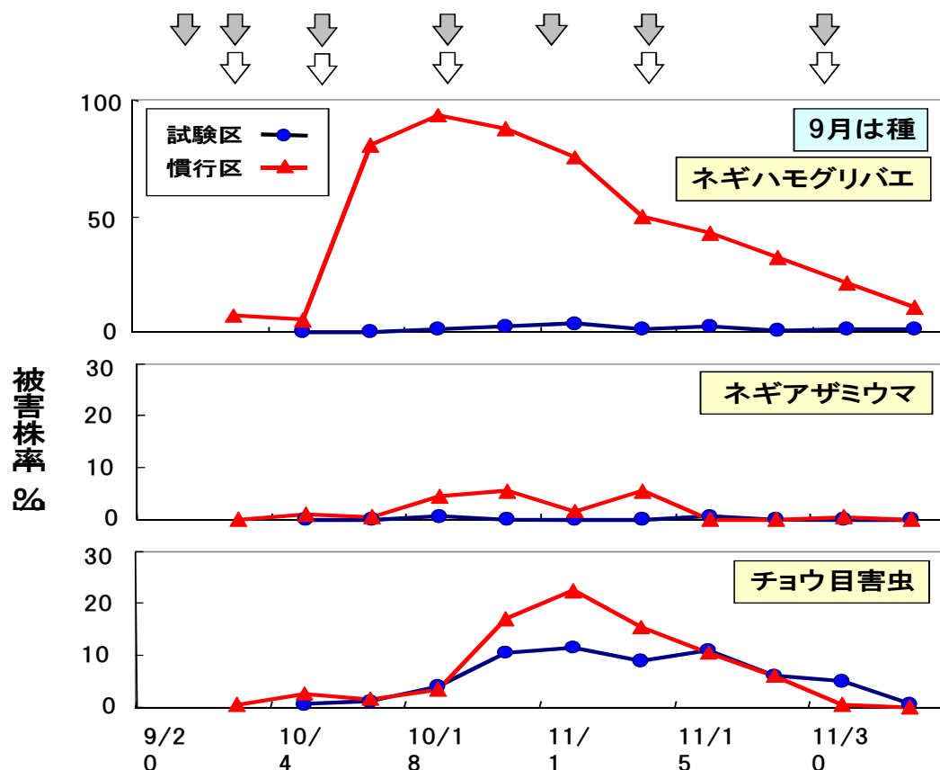
図4 ネギハモグリバエ（上段）とネギアザミウマ（中段）、チョウ目害虫（下段）に対するUV除去フィルムの防除効果（2007年9月は種、12月収穫）年6月は種、8月収穫）
