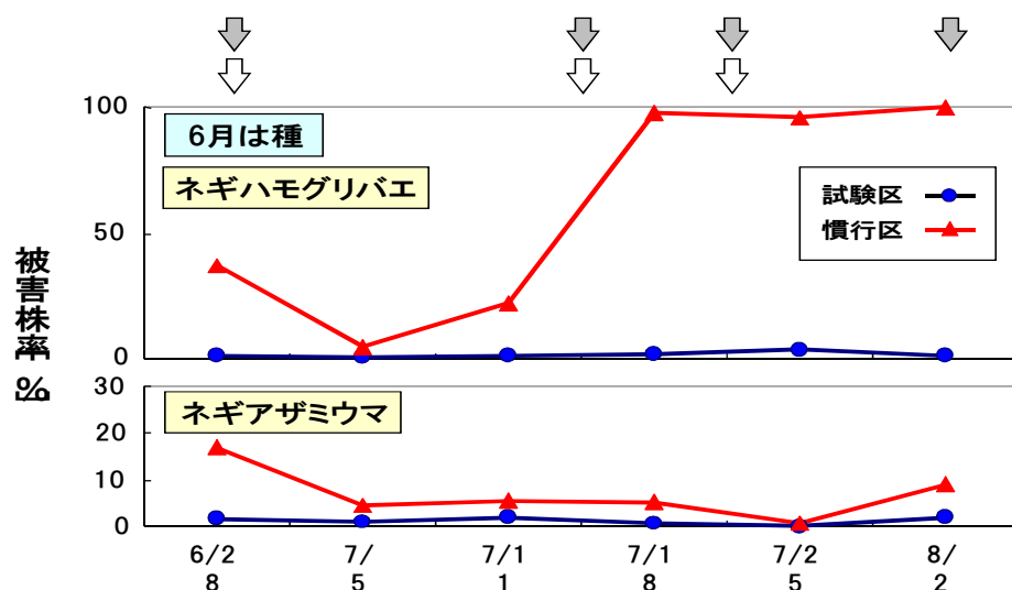
図3 ネギハモグリバエ（上段）とネギアザミウマ（下段）に対するUV除去フィルムの防除効果（2007年6月は種、8月収穫）
