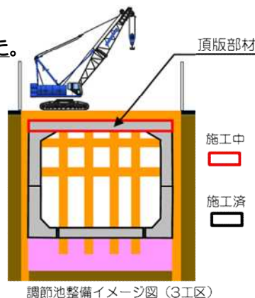
調節池整備イメージ図（3工区）
