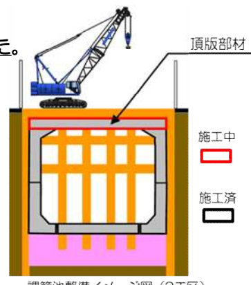
調節池整備イメージ図（3工区）
