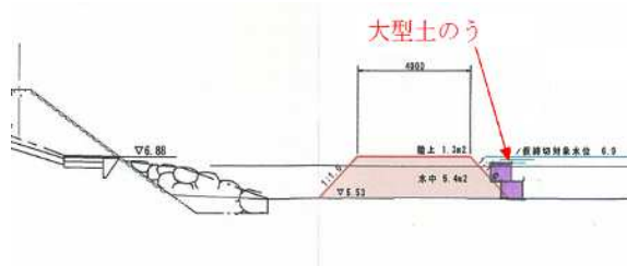
標準断面図
