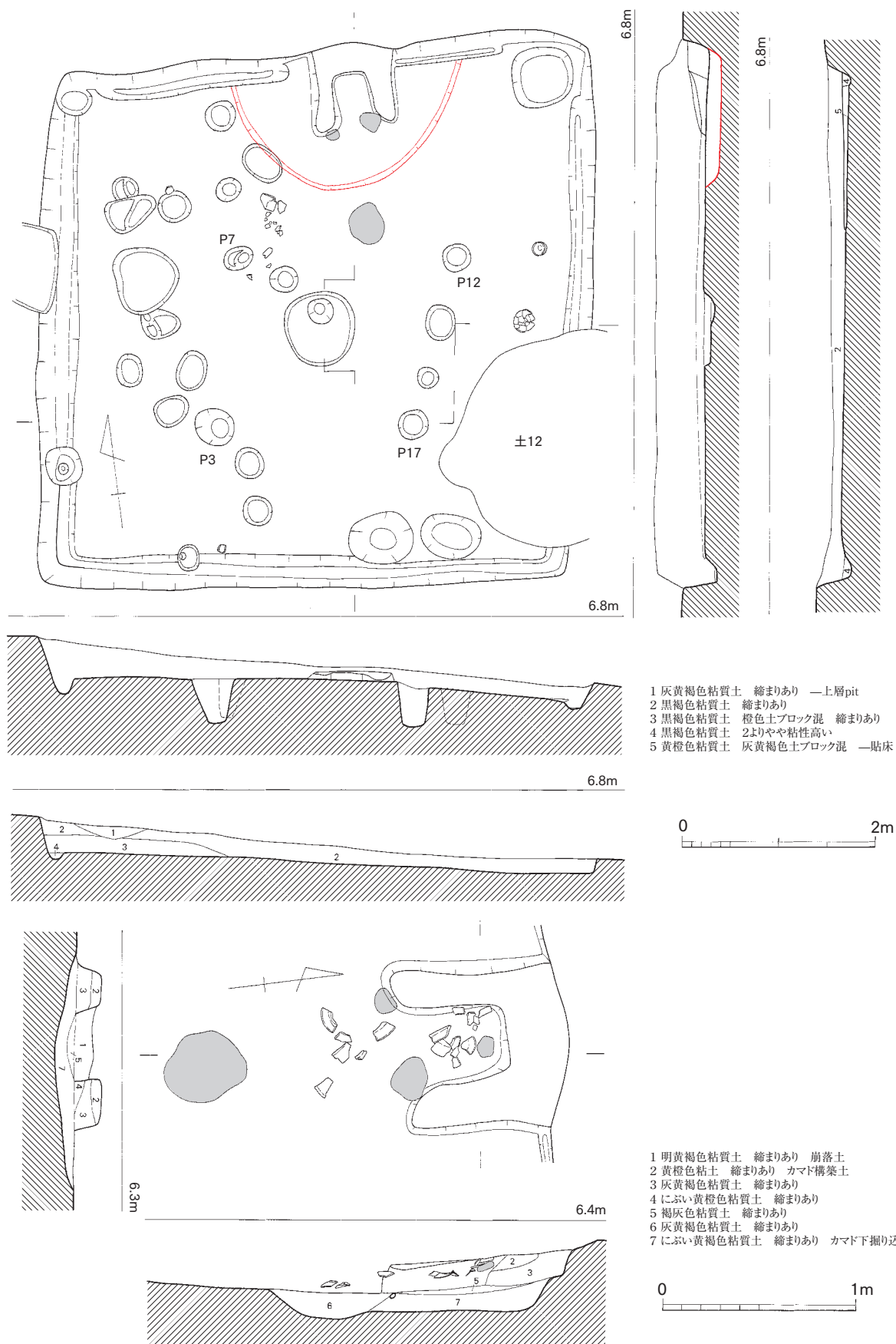
第37図 27号竪穴住居跡実測図 (1/60、1/30)
