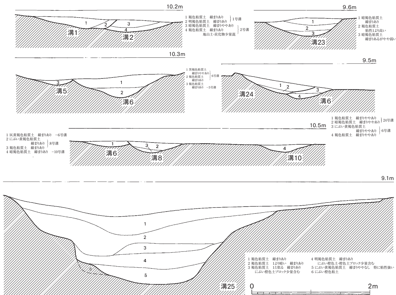
第63図 溝1・2・5・6・8・10・23～25土層実測図(1/40)
