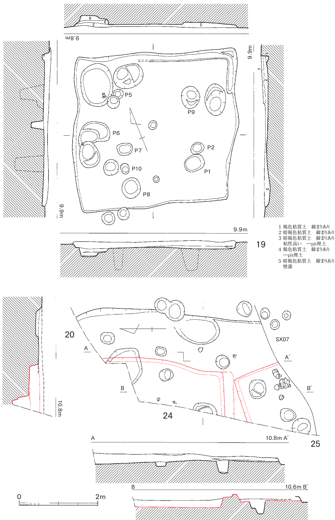
第31図 19・20・24・25号竪穴住居跡実測図 (1/60)
