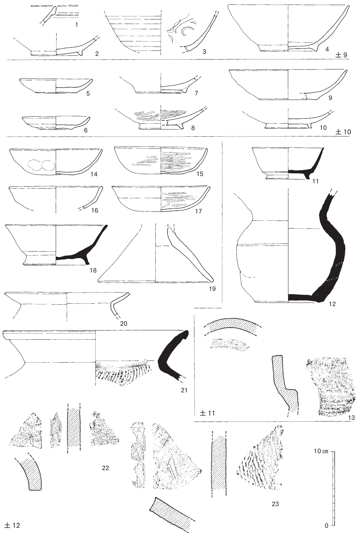
第58図 9～12号土坑出土土器実測図 (1/3)
