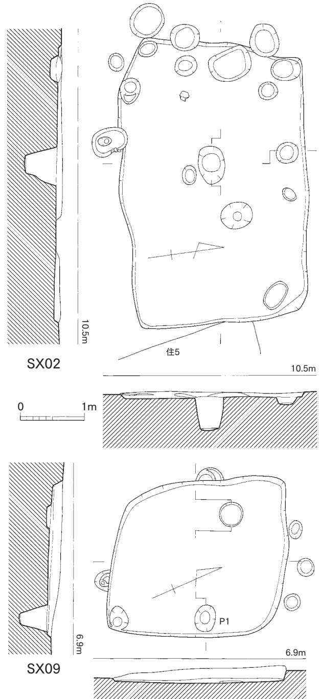
第41図 SX02・09実測図 (1/60)
