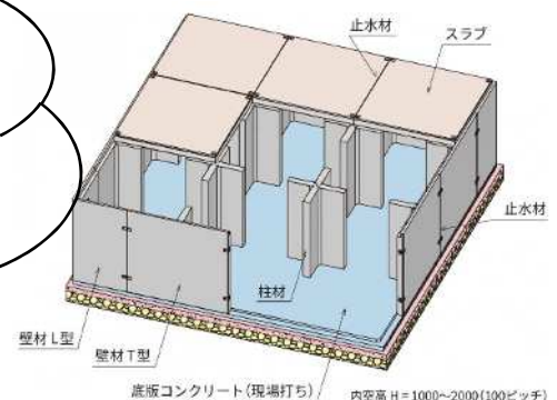
(調節池構造イメージ)
