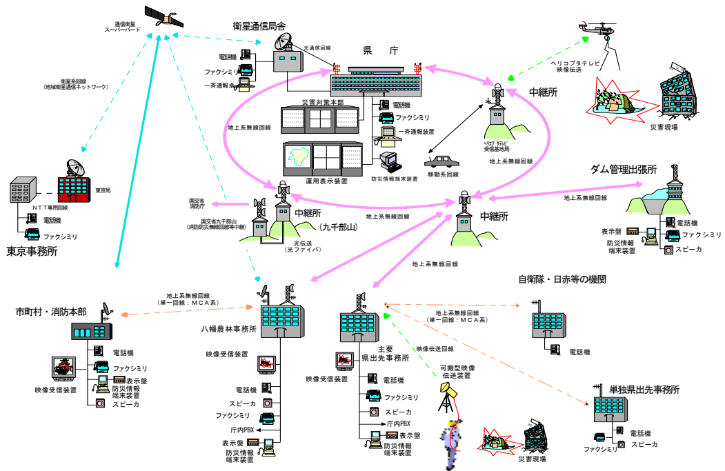
福岡県防災・行政情報通信ネットワーク（ふくおかハイパーネット）概念図
