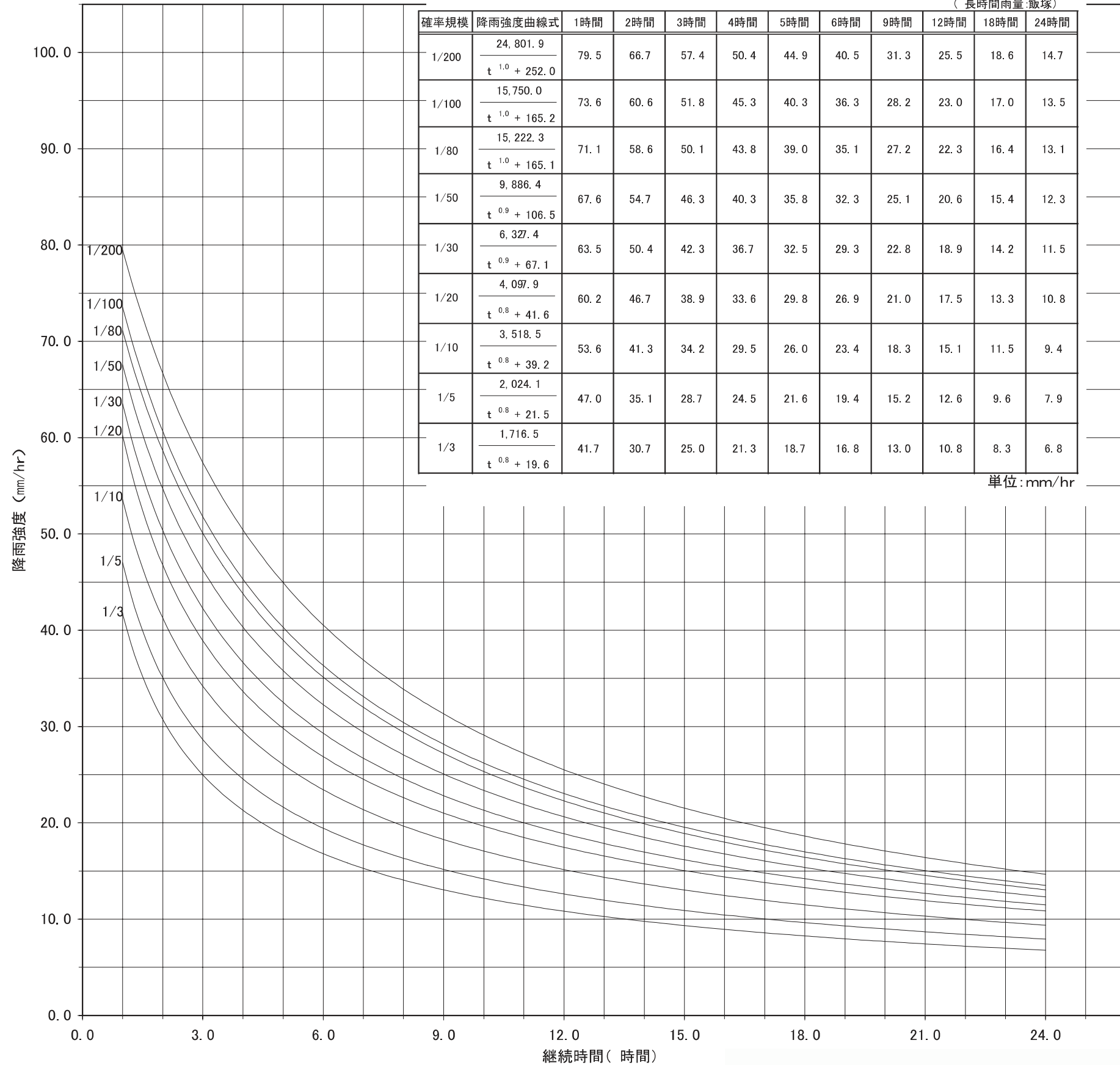
長時間降雨強度曲線式 飯塚(气象台)
