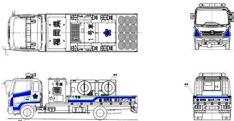
見取図
