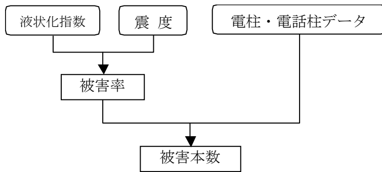
図 4.3-1 電柱・電話柱被害の想定の流れ
