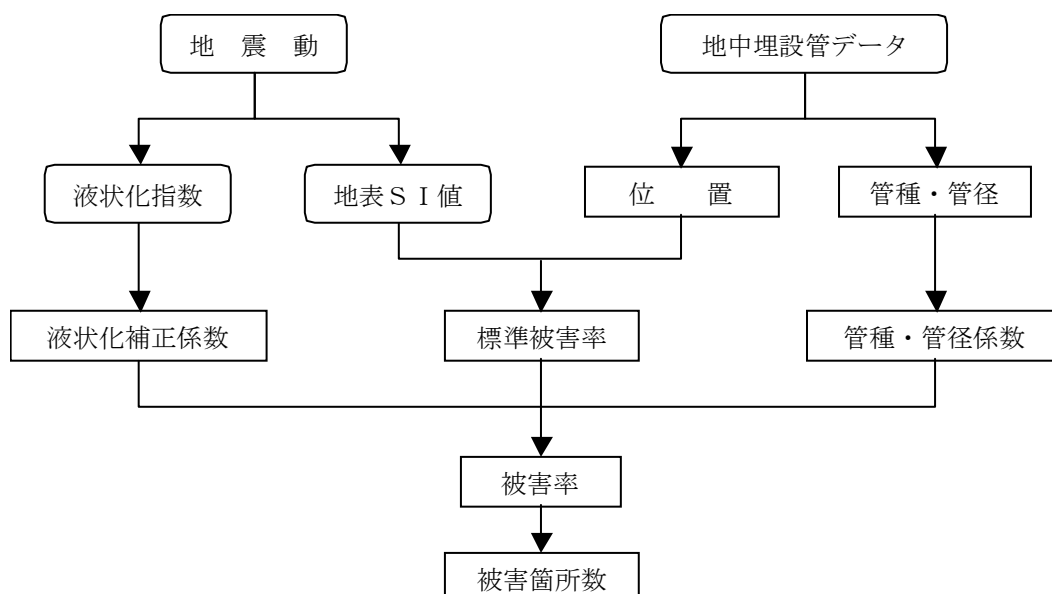
図 4.1-1 地中埋設管被害の想定の流れ
