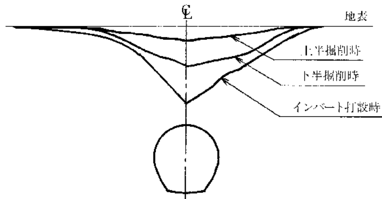
図一24 地表沈下分布図
