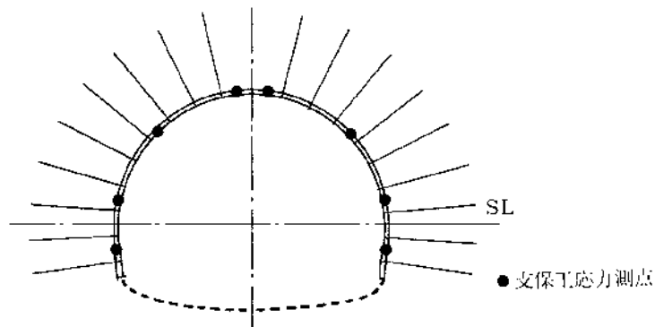
図一25 鋼製支保工測点配置図
