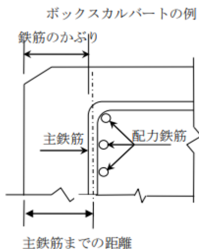
図 3-9-1 鉄筋のかぶり
