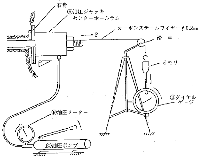
図4-3 引抜試験概要図
