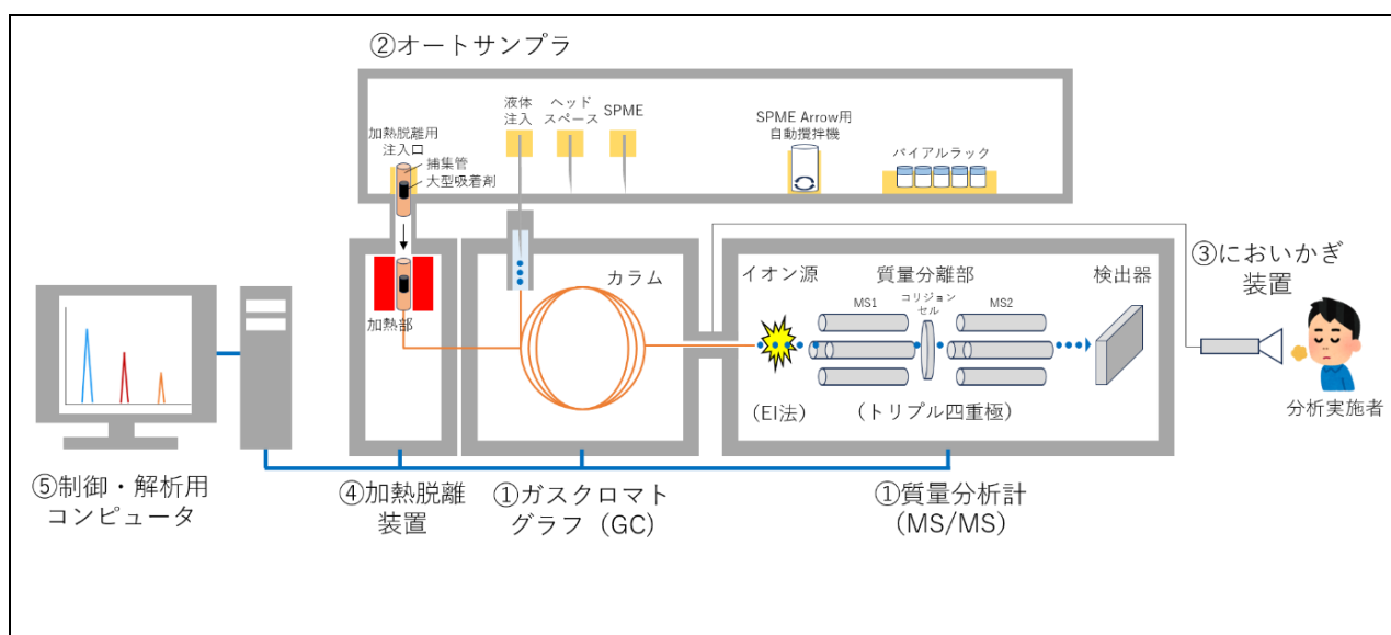
図1 食品成分分析装置の構成概略図
