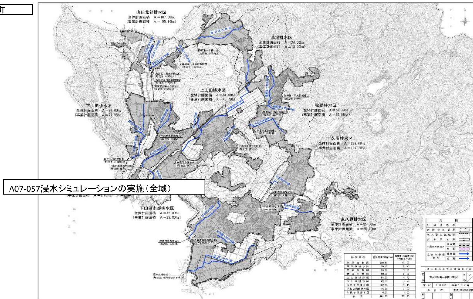
図 1.2 下水道計画一般図(雨水)
