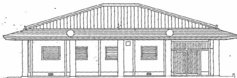
立面図(西側)
