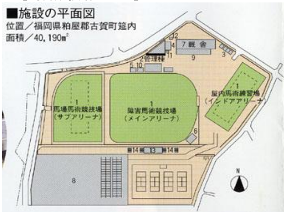
【馬術競技場平面図】
