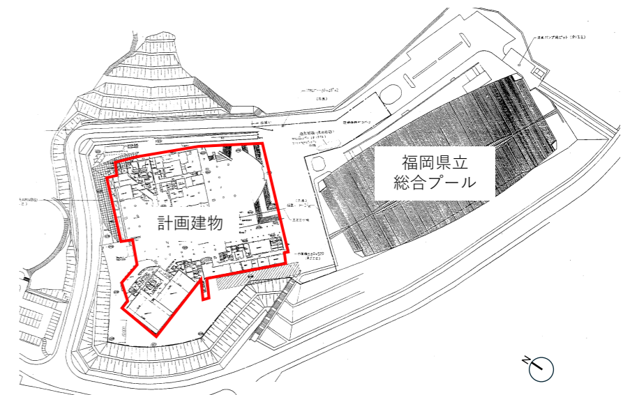
配置図
