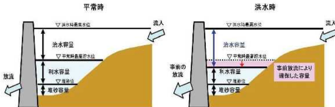
洪水前目標水位H事前放流の設定
