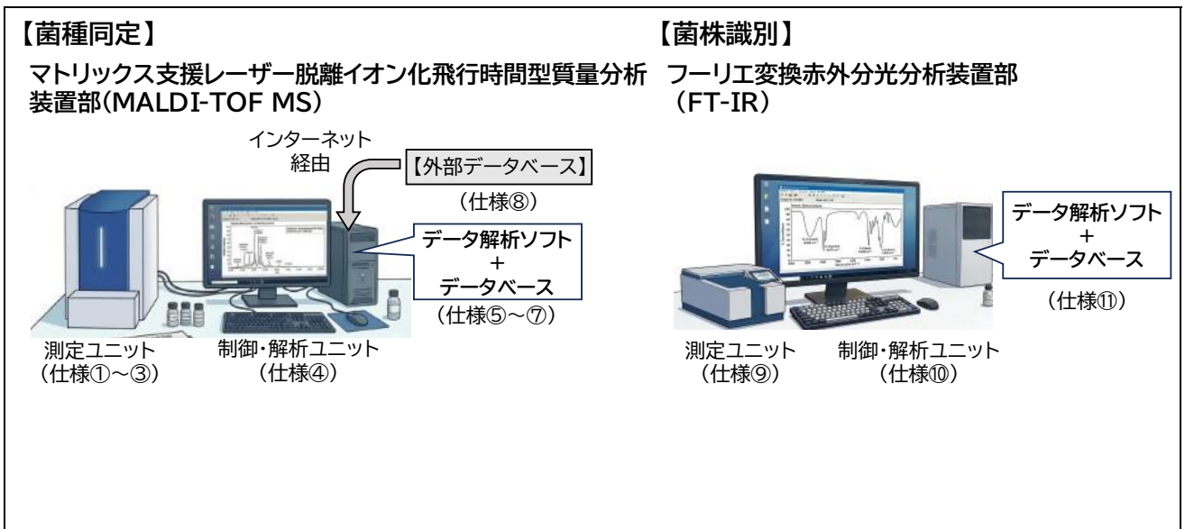
図1 微生物迅速同定装置の構成概略図
