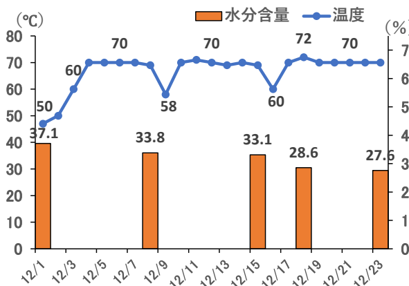
枝葉チップの発酵状況
