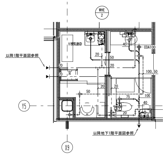
1階 キッズスペースWC、1F授乳室②詳細図 S=1:50
