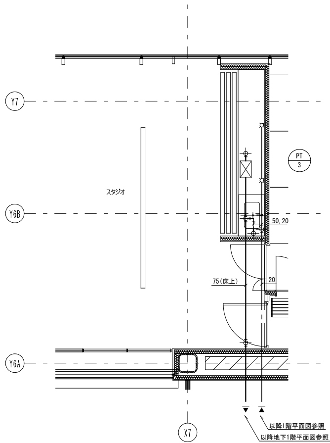
1階 スタジオ詳細図 S=1:50
