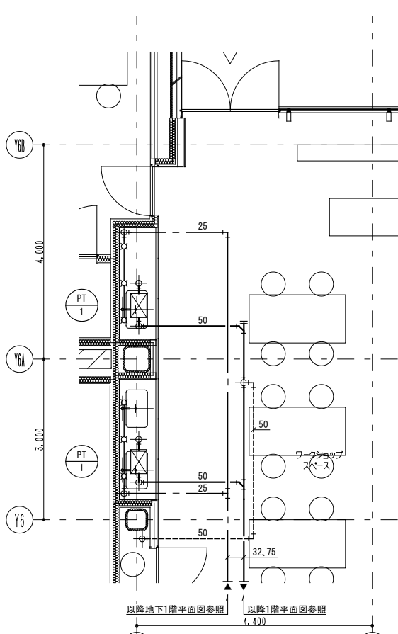
1階 WC①(BOH)、1F倉庫F詳細図 S=1:50
