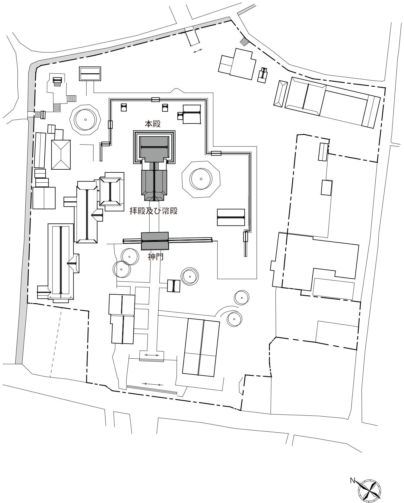
図2 宇美八幡宮配置図 縮尺 1/1,000
