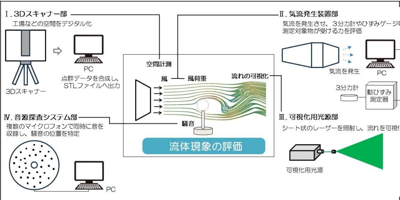
装置構成概略図
