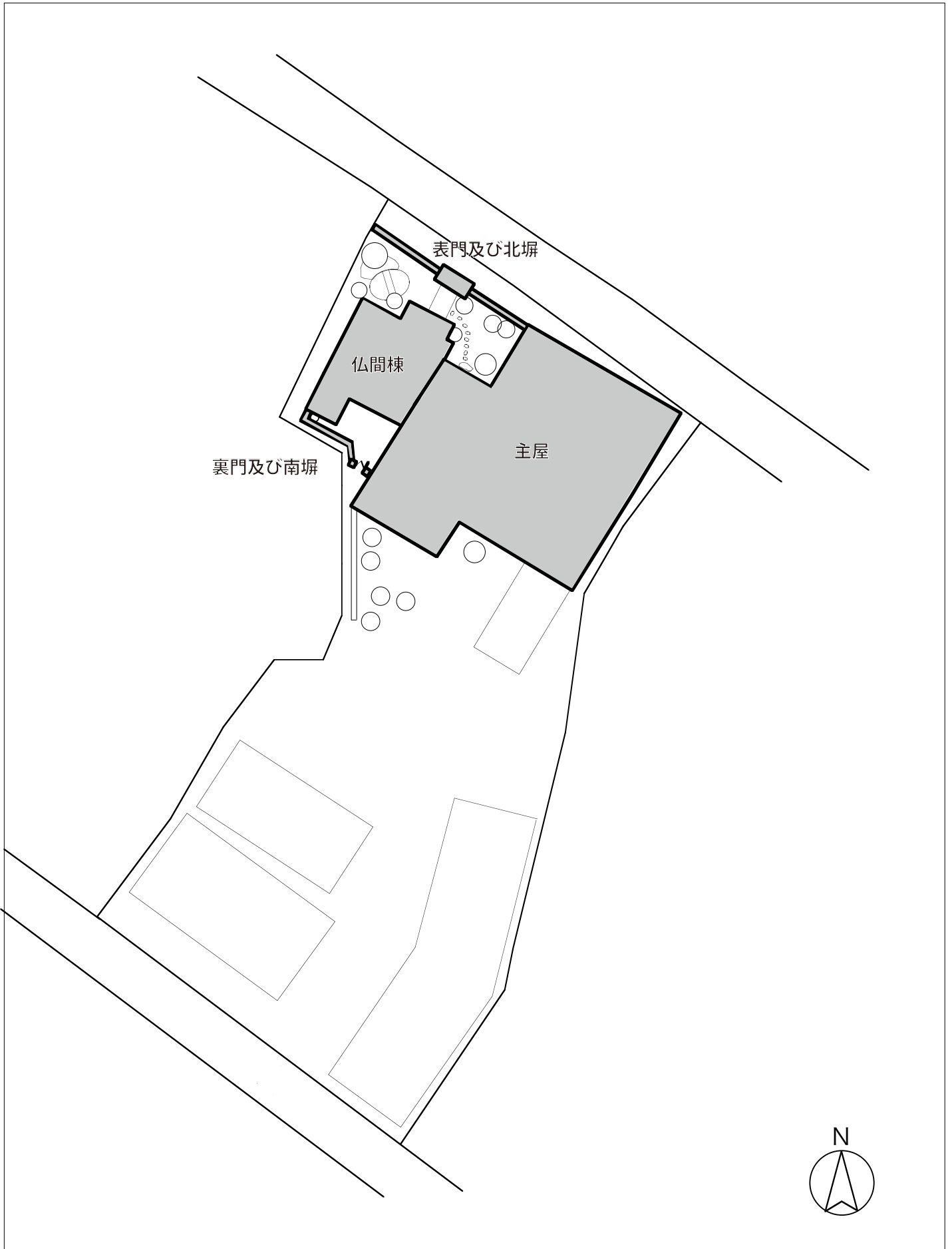
図2 森田家住宅配置図
