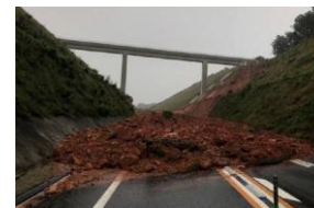
暫定2車線区間における被災状況
