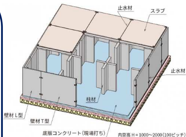
※調節池構造イメージ
