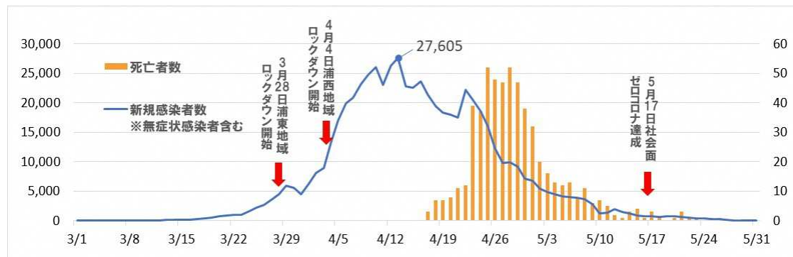
(表1) 上海市感染者数等推移 (出典) 上海市政府資料を基に上海事務所作成
