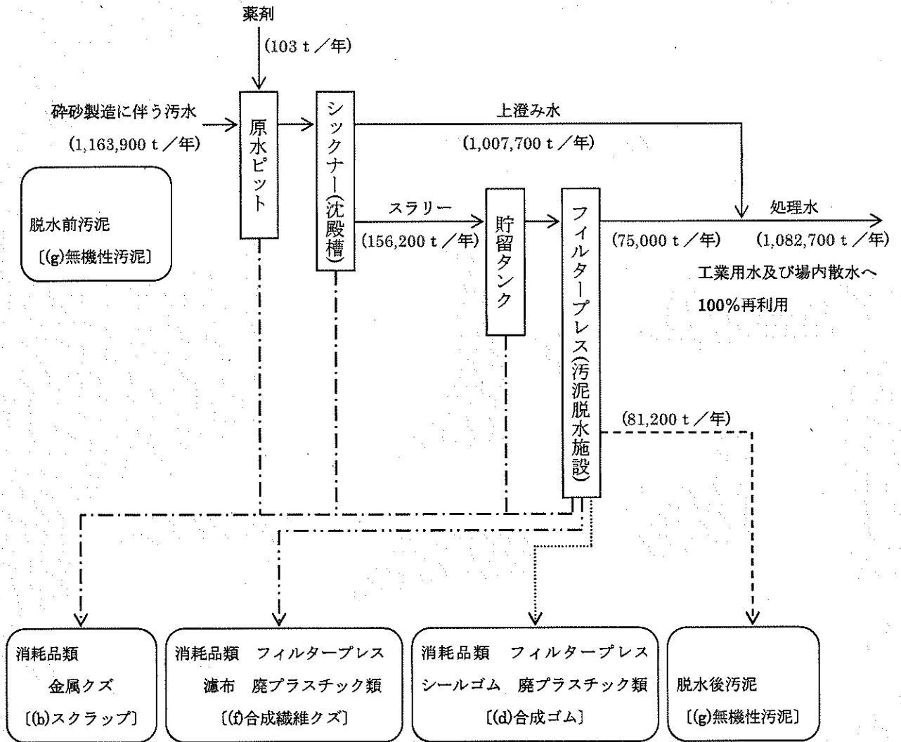
図5 汚水処理フローシート [No. 5]
