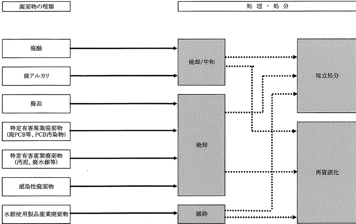
(表1) 廃棄物処理フローシート (廃棄物の処理法)
