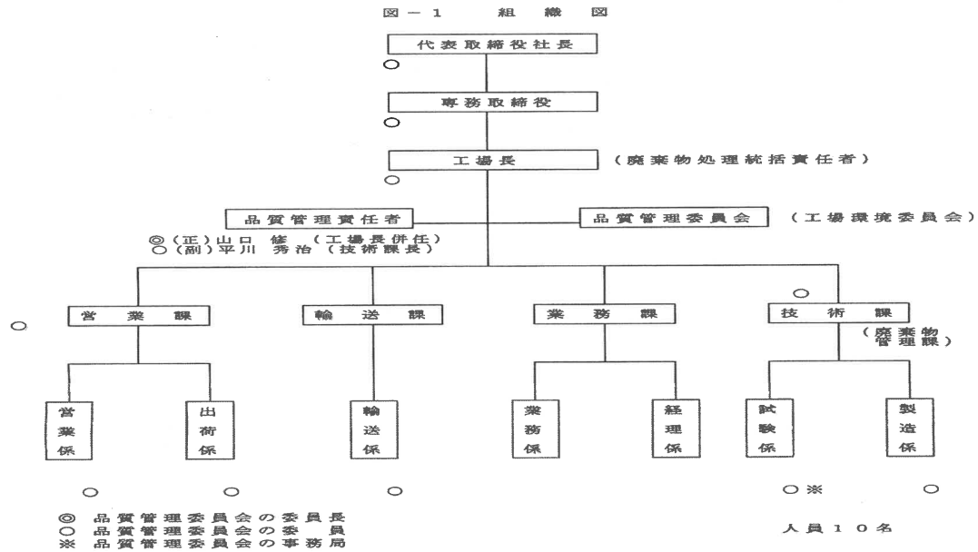
(管理体制図)
